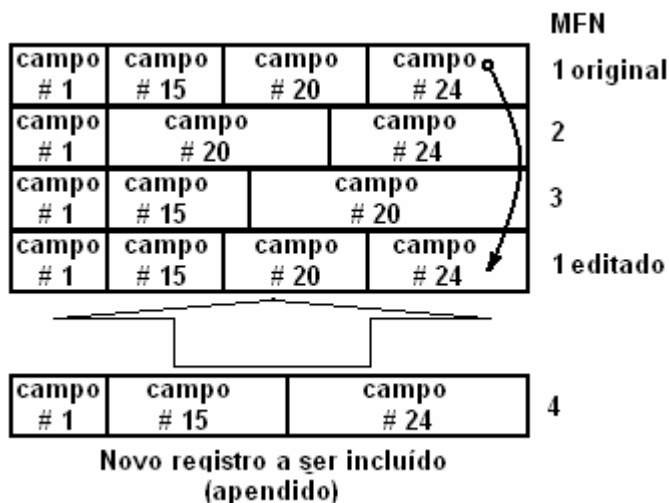
Figura-3: Base de Dados durante sua operação
