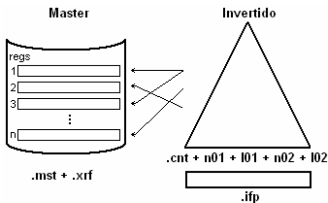
Figura-2: Composição de Base de Dados CDS/ISIS em arquivos
